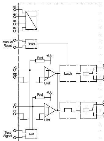
ELMON rail 34 Prinzipschaltbild / Simplified diagram
