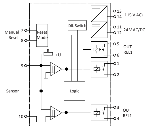
Prinzipschaltbild / Simplified diagram
